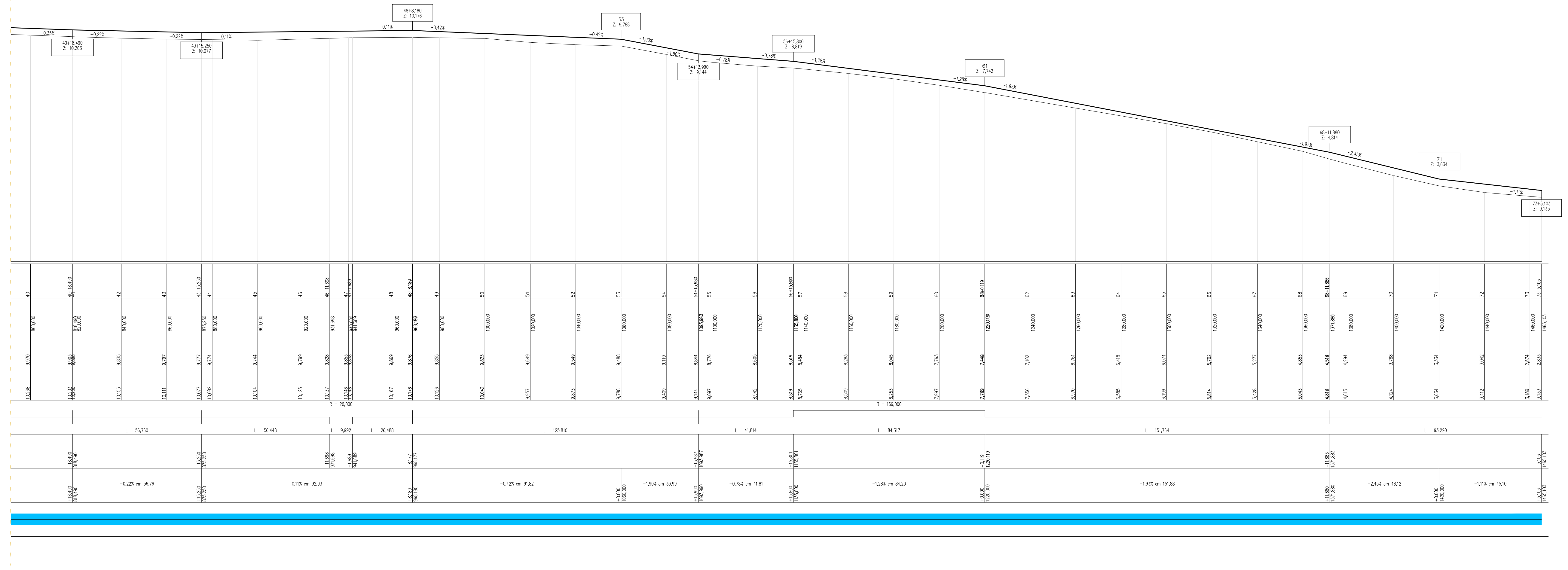
PERFIL DO RAMAL VILA SAO MIGUEL Escala 1:1000
