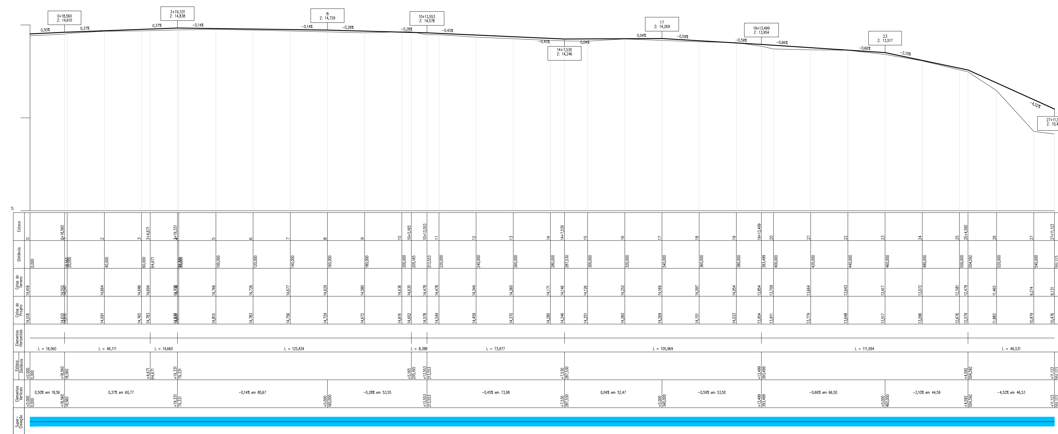
PERFIL DA RUA DOMINGOS FERNANDES-T1 Escala 1/1200
