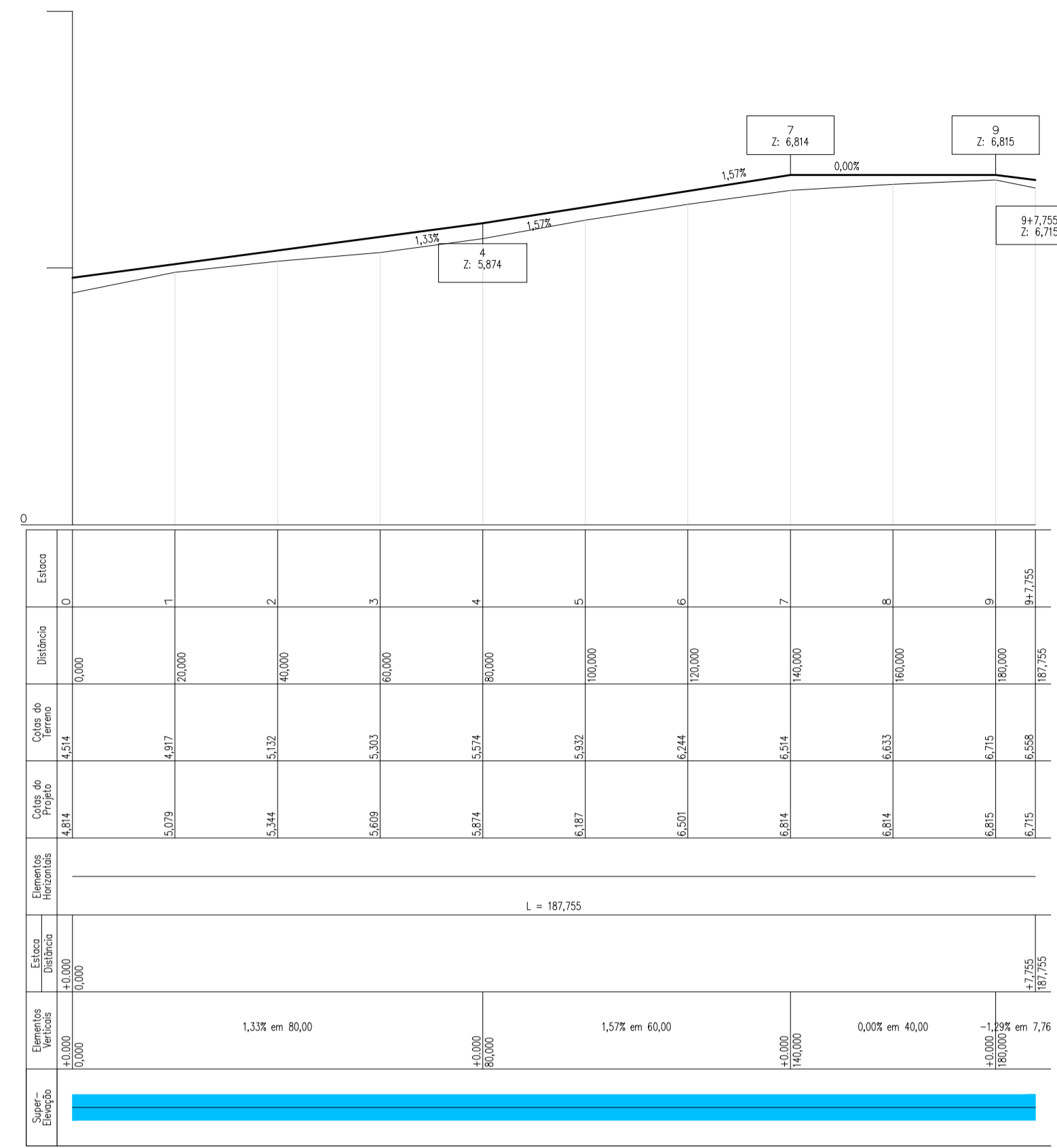
PERFIL DO RAMAL 2 Escala 1/1200
