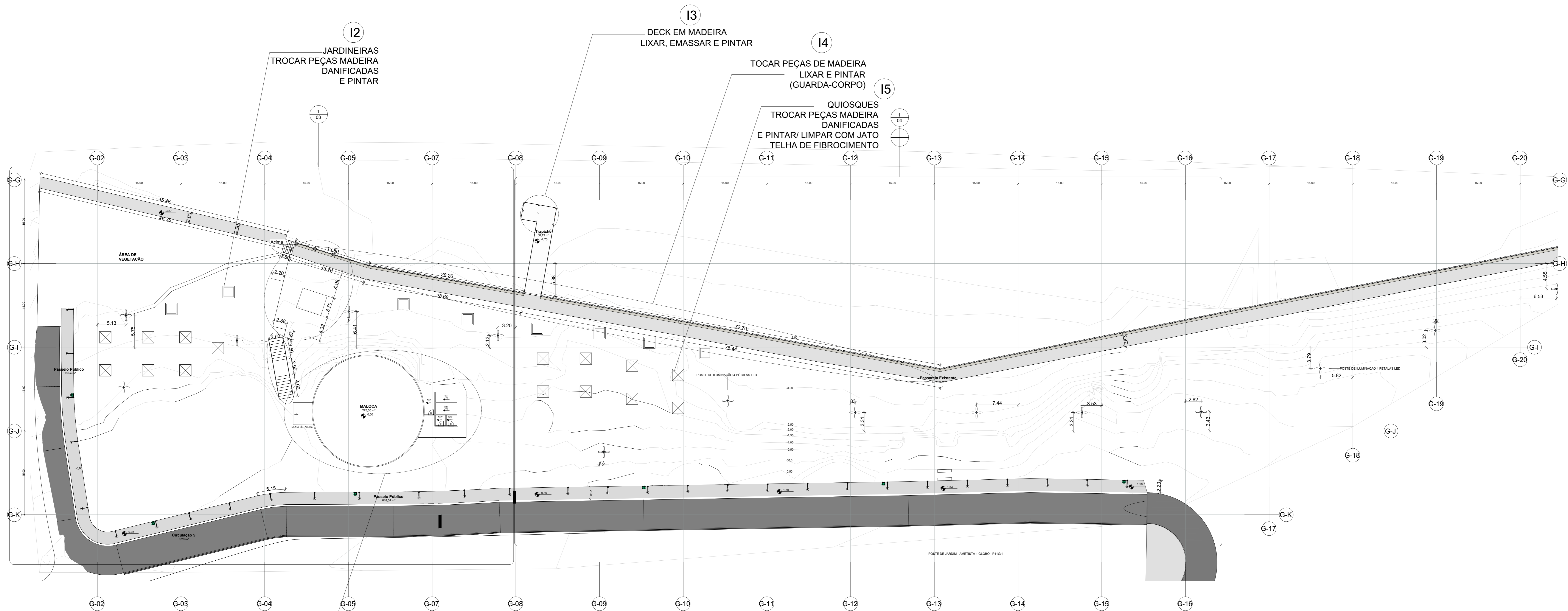
PLANTA BAIXA DE INTERVENÇÕES 1:100
