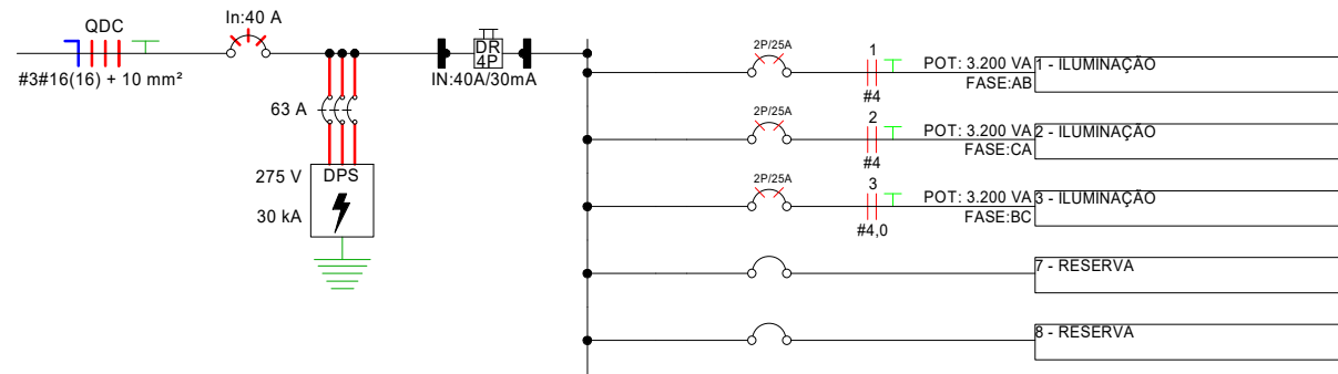
Diagrama Unifilar - QDC
