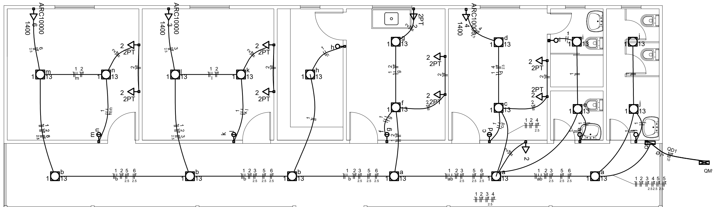
PLANTA BAIXA Escala 1/50
