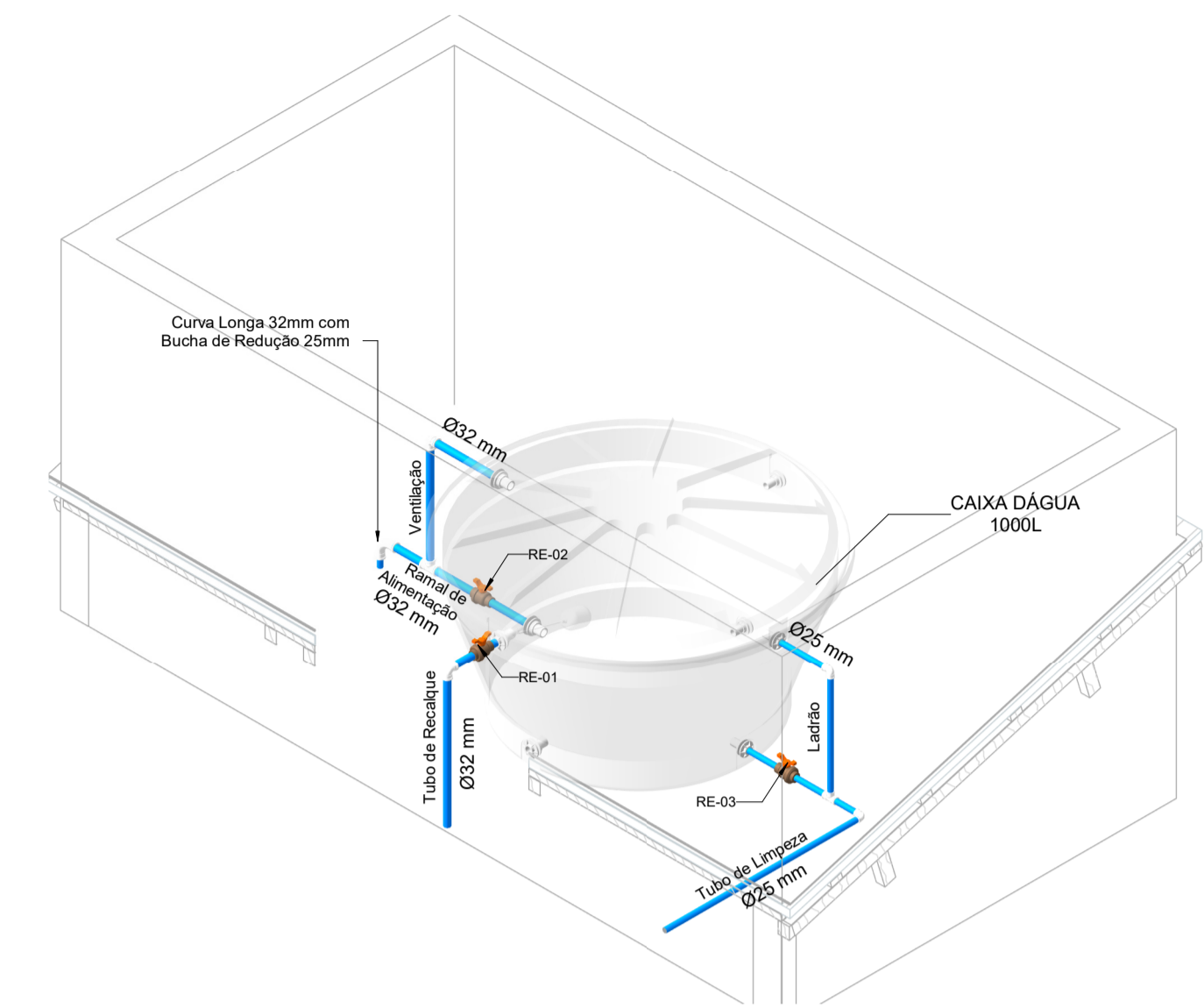
4 ISOMETRIA CAIXA D'ÁGUA
