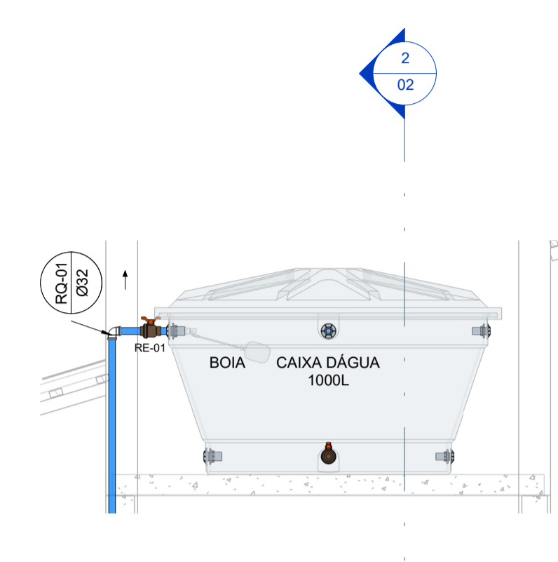
3 CORTE 02 CAIXA D'ÁGUA 1:25
