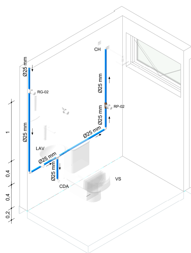
5 ISOMETRIA BHO M. E F.
