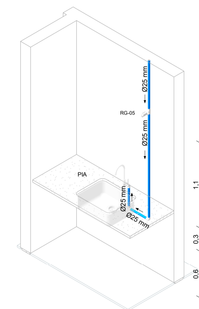
7 ISOMETRIA PIAS - COPA E CONSULTÓRIOS
