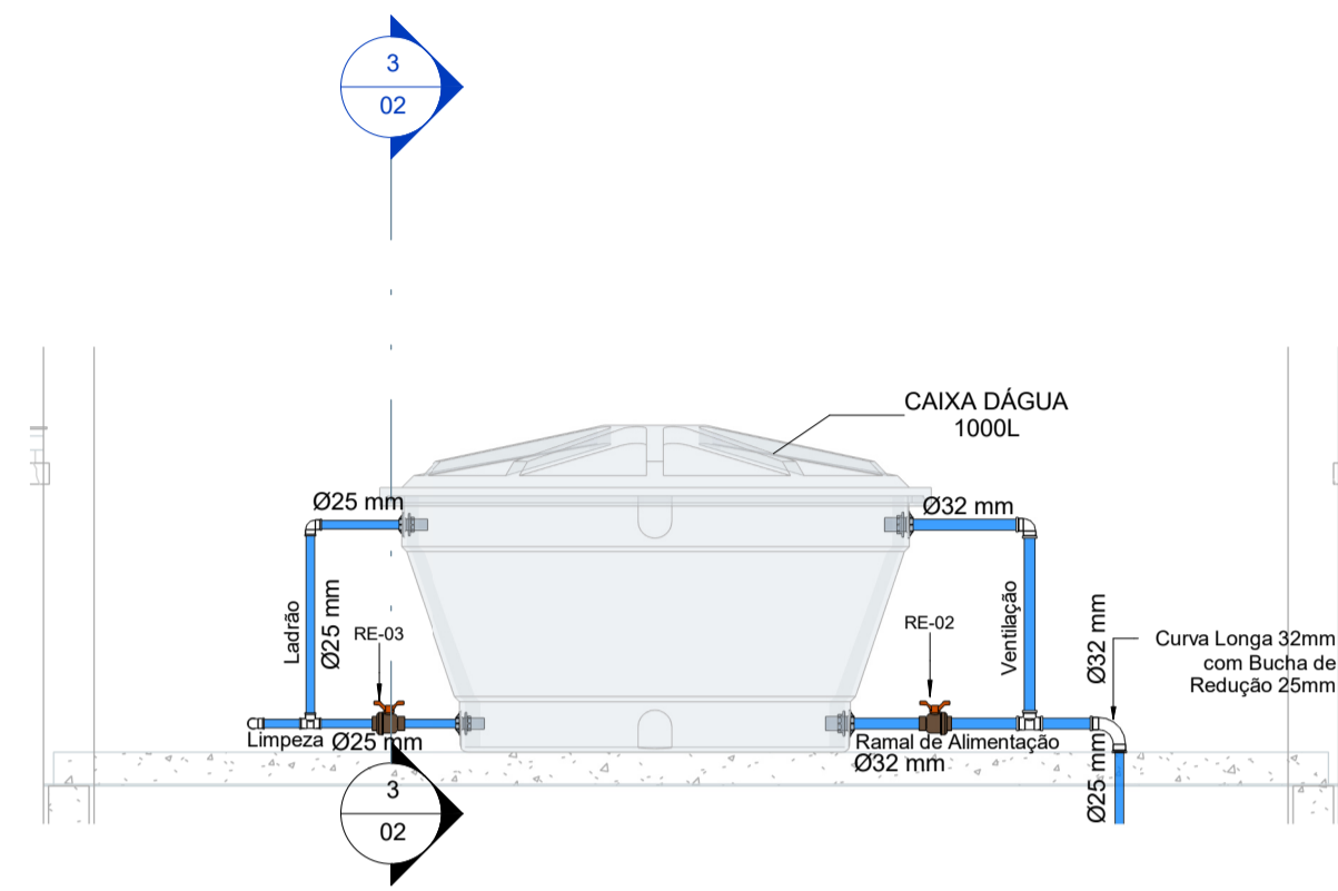
2 CORTE 01 CAIXA D'ÁGUA 1:25
