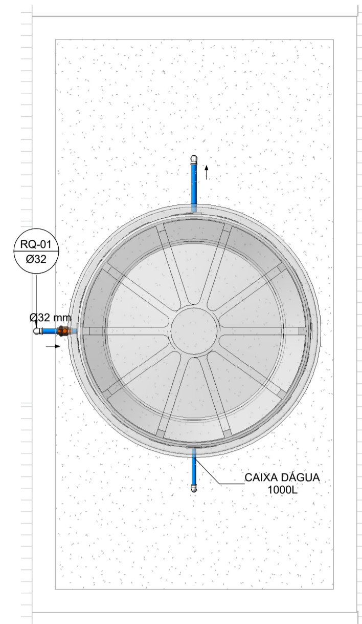
1 DET - CAIXA D'ÁGUA 1:25
