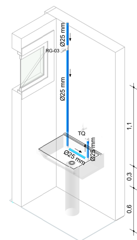
6 ISOMETRIA TANQUES
