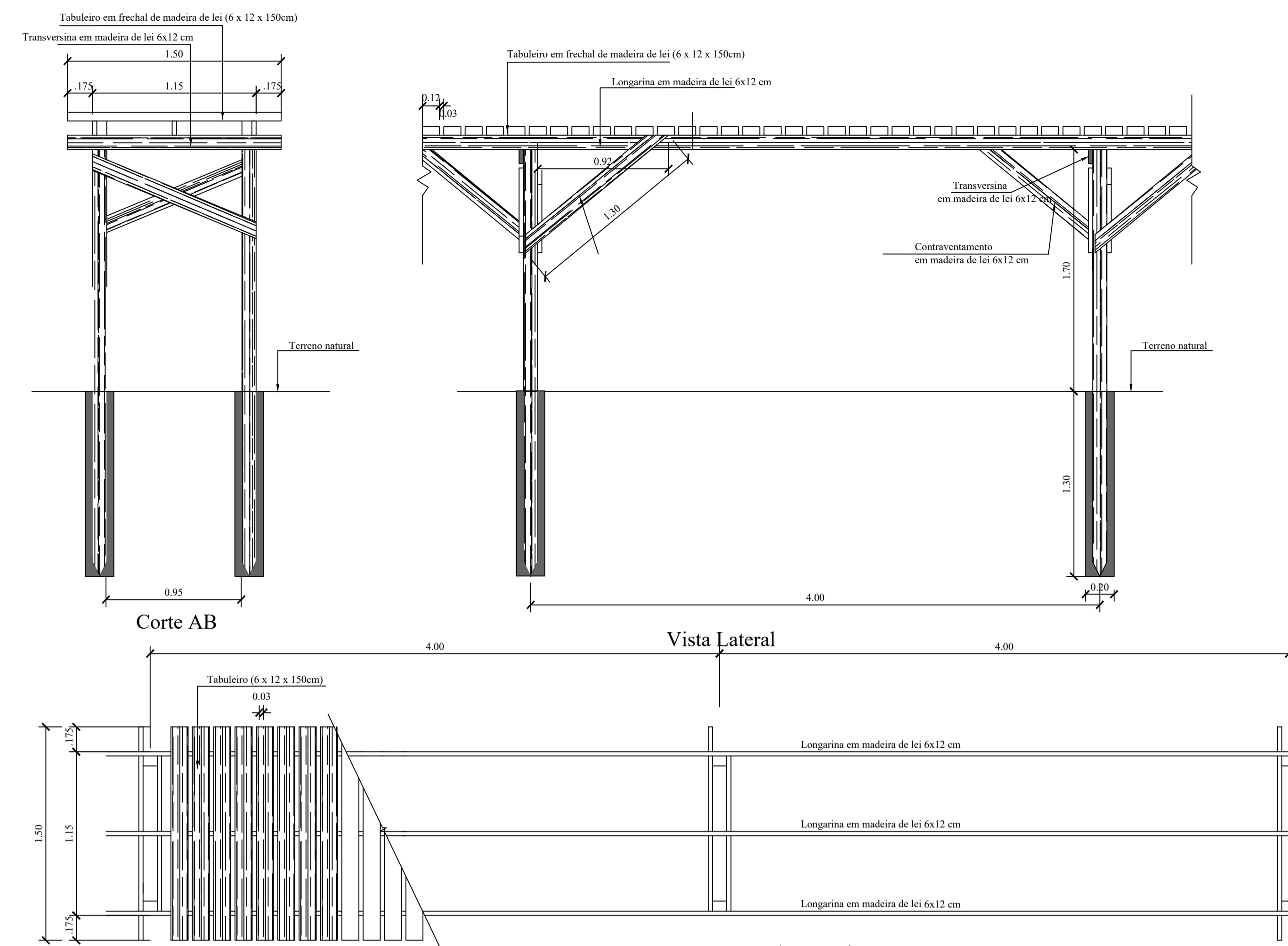
DETALHE- PASSARELA DE 1,50 M
