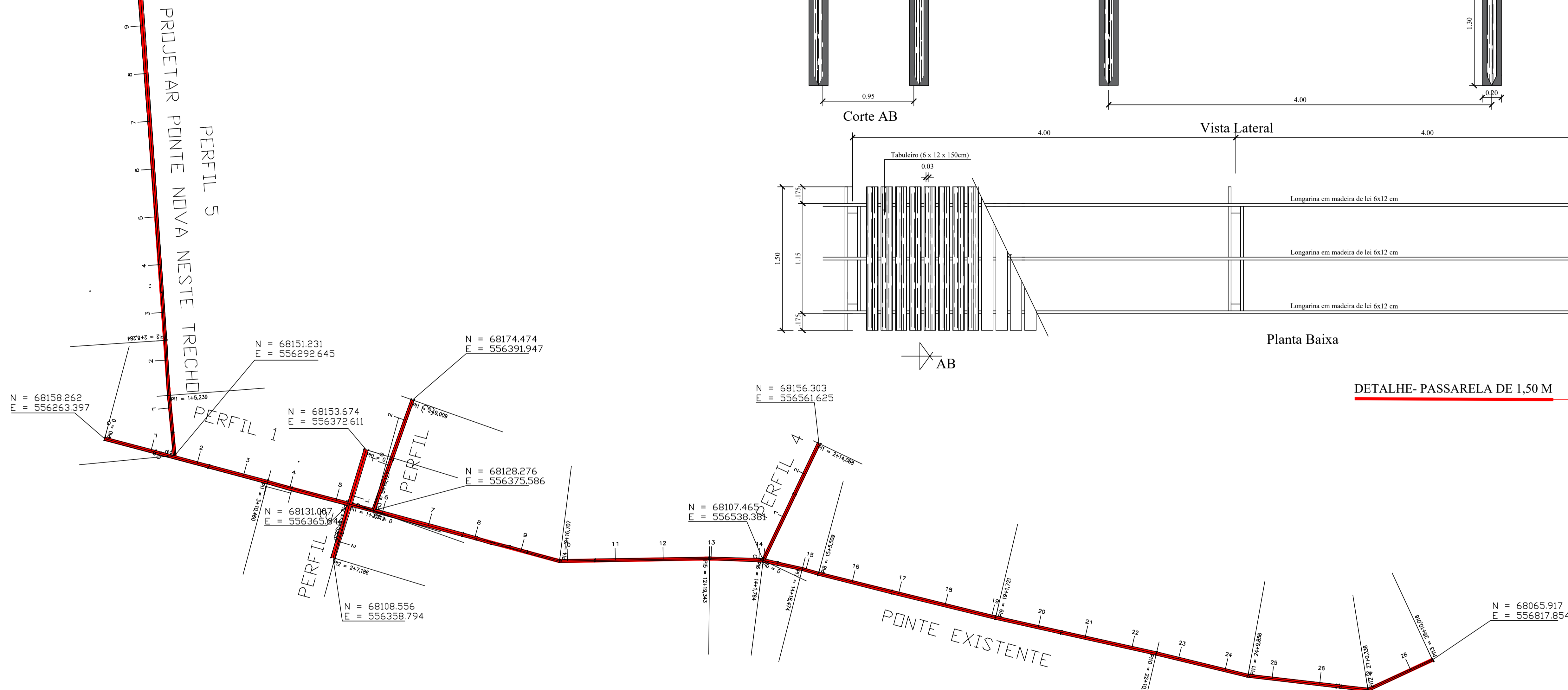
MUNICÍPIO DE ITAUBAL PLANTA BAIXA ESC.:1:1000
