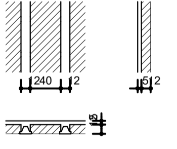
Detalhe 2 (esc. 1:50)
