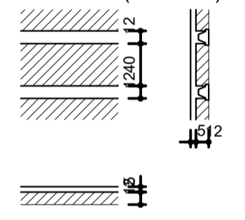
Detalhe 2 (esc. 1:50)
