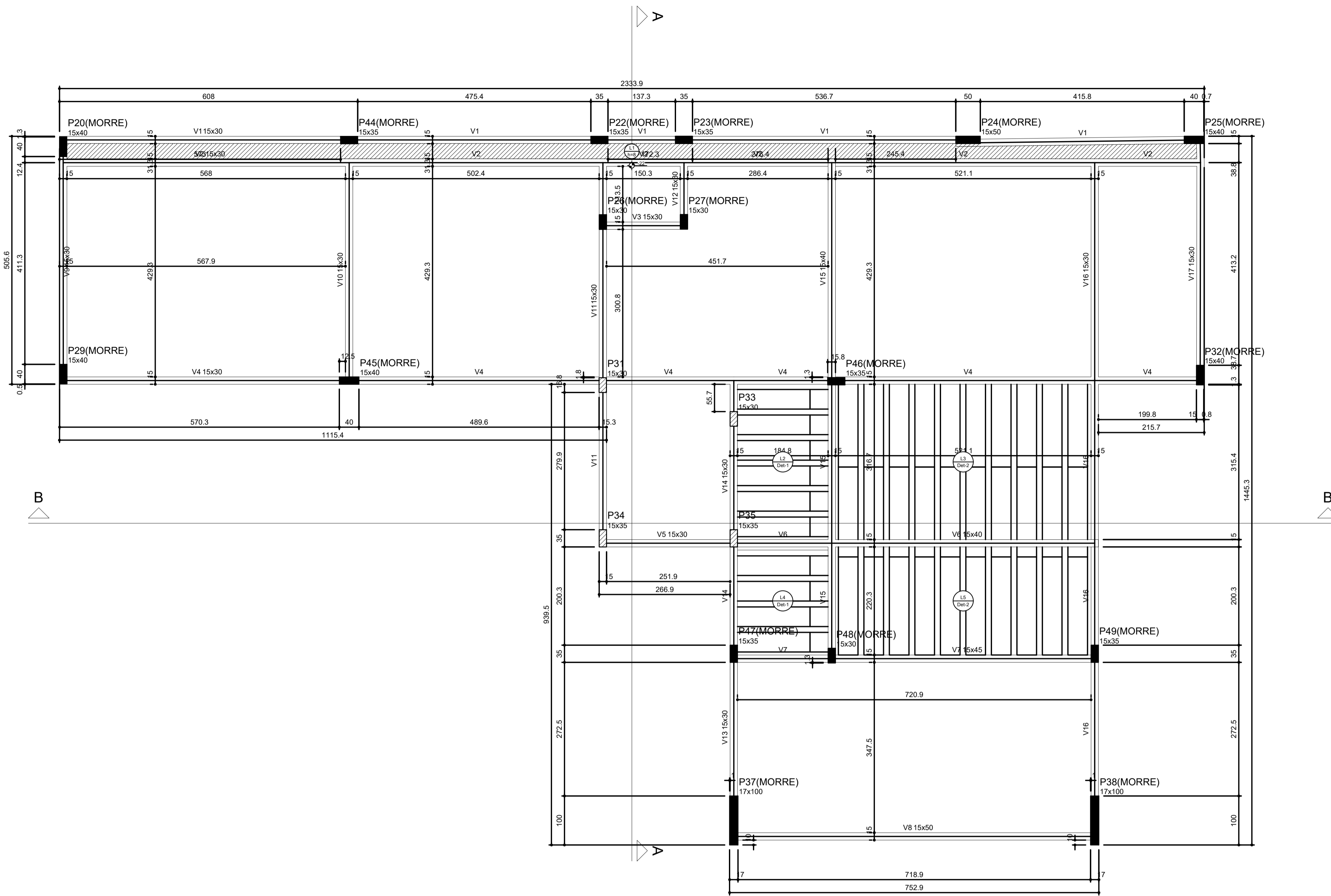
Forma do pavimento Cobertura (Nível 660) escala 1:50
